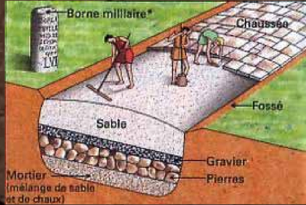
Détail de construction d'une voie romaine
