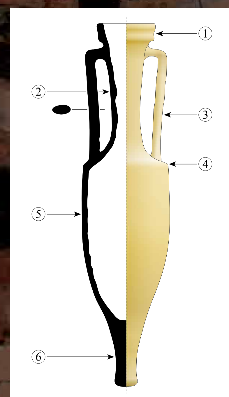
Coupe d'une amphore vinaire de type Dressel 1B. Contenance d'environ 26 litres.
